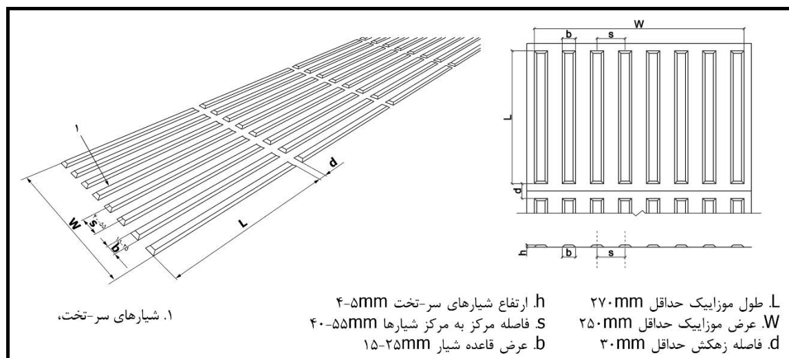
شکل ۷-۲- چیدمان، فواصل و ابعاد کفپوش شیاردار سر-تخت
