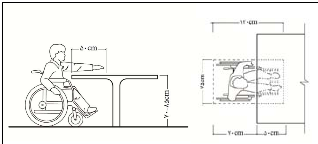
شکل ۲-۳۲- ابعاد میز
