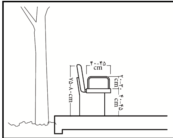
شکل ۲-۳۱- ابعاد نیمکت
