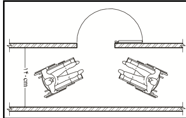
شکل ۲-۳- حداقل عرض راهرو
