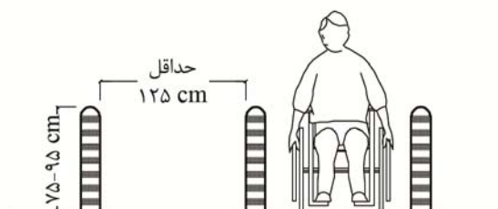
شکل ۲-۱۱- ابعاد و فاصله بین دو میله هدایت‌کننده
