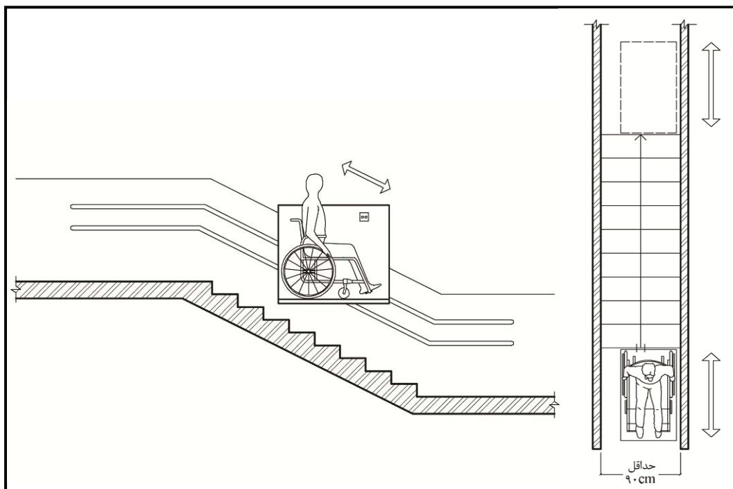
شکل ۳-۱۶- بالابر جانبی
