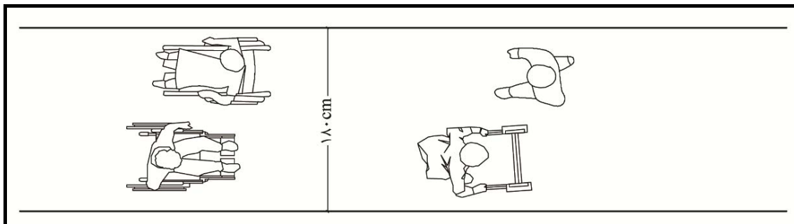
شکل ۲-۲- حداقل عرض مفید پیاده‌رو پرتردد
